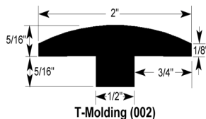
T-Molding (002)
