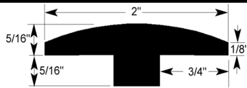
T-Molding (002)
